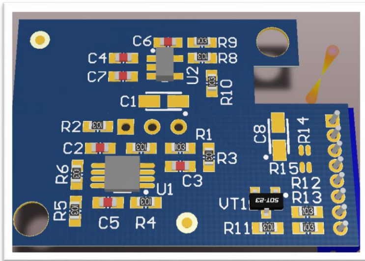
Схема 7. Плата SC-FIS-M
