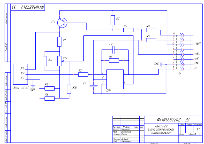
Схема 8. Электрическая схема ТК-М
